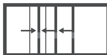
Coulissants 3 vantaux 3 rails, ouverture 2/3 et jusqu'à 6 vantaux
