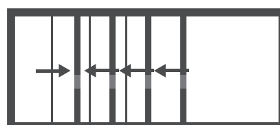
Coulissants 4 vantaux 4 rails, ouverture 3/4 et jusqu'à 8 vantaux
