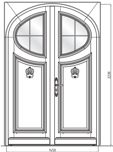
Plan filaire dessiné par Bel'M, selon l'esquisse du client.
