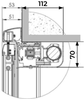
Motorisation SIB - Automatisme pour volet coulissant
