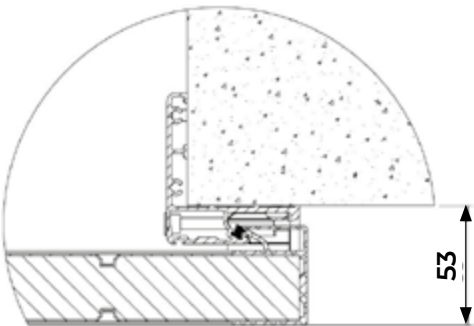
COUPE HORIZONTALE - VANTAIL FERMÉ
