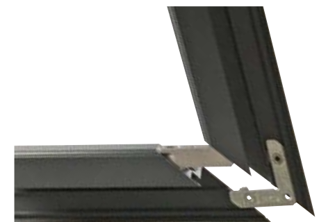
2 équerres d'assemblage pour le dormant précadre
