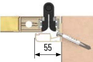
Pose entre tableaux
