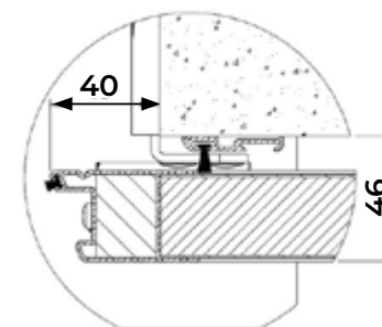
COUPE VANTAUX JUMELÉS - 2 VANTAUX OUVERTS
