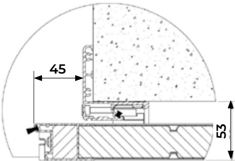
COUPE HORIZONTALE - VANTAIL OUVERT
