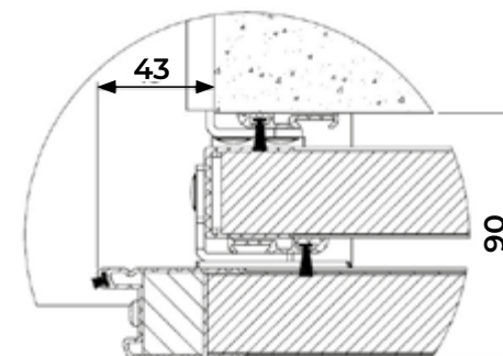
COUPE VANTAUX JUMELÉS - 2 VANTAUX OUVERTS
